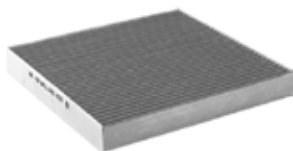
AFC8023 A: 211 B: 198 C: 25 D: OEM : 4293145 BRILLIANCE H220
